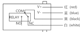
出线定义
