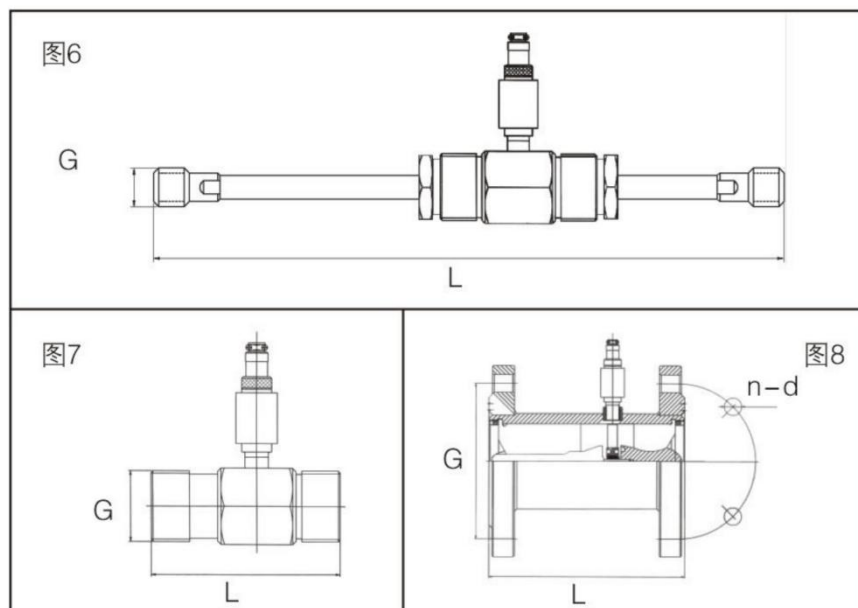
图6 WLL-102-4~10传感器结构及安装尺寸示意图
