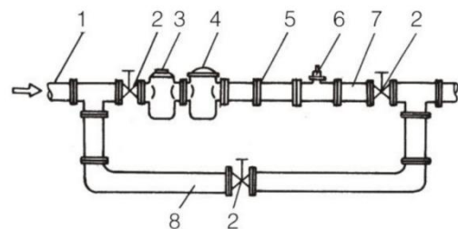
1-入口； 2-阀门； 3-过滤器； 4-消气器； 5-前直管段； 6-传感器； 7-后直管段； 8-旁路
